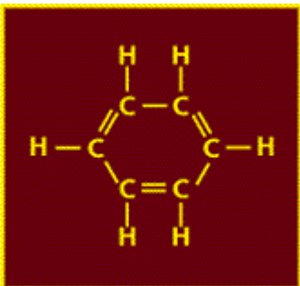
Benzene ring
